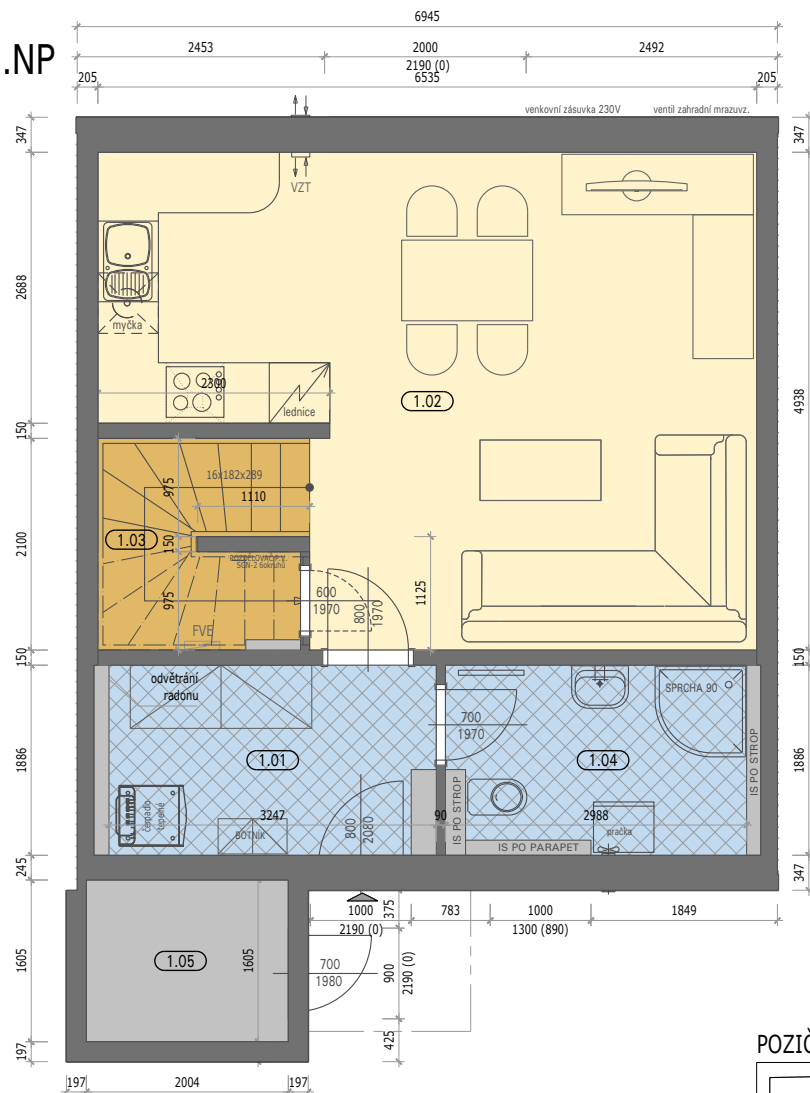
LEGENDA MÍSTNOSTI 1.NP
